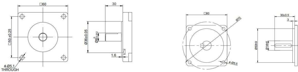
NEMA 24
