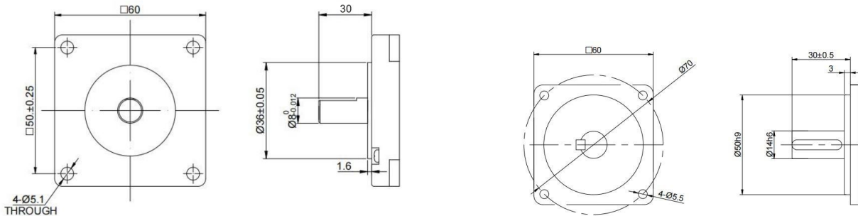
NEMA 24
